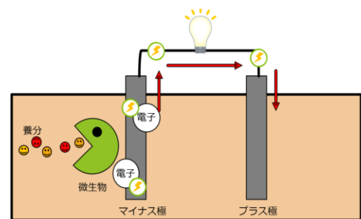
微生物燃料電池のしくみ
